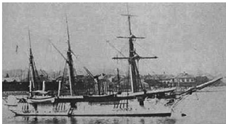
El Iltis , cañonero de casco de hierro construido en Dantzing en 1878, que fue enviado al Pacífico en 1881. Desplazaba 412 toneladas y se propulsaba mediante una máquina de 250 caballos que la permitía navegar a una velocidad máxima de 10 nudos. Su tripulación estaba formada por 85 hombres entre oficiales y marinería y poseía como armamento dos cañones de 125 mm y dos de 87 mm
